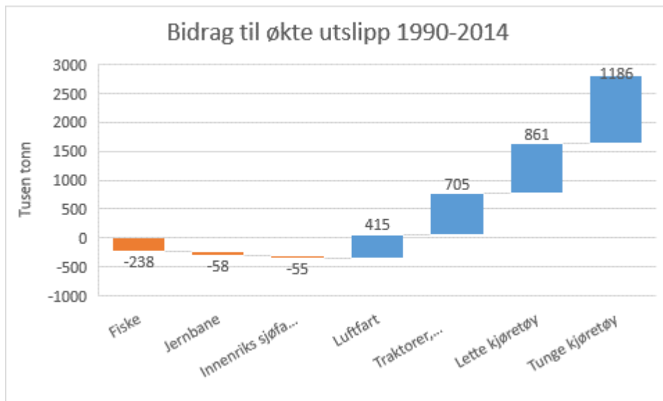
Figur 13: Utslippsøkningen i antall tonn siden 1990 har vært størst for tungtrafikken, men lette kjøretøy – varebiler – har også vært en viktig kilde til økte utslipp. Kilde SSB
