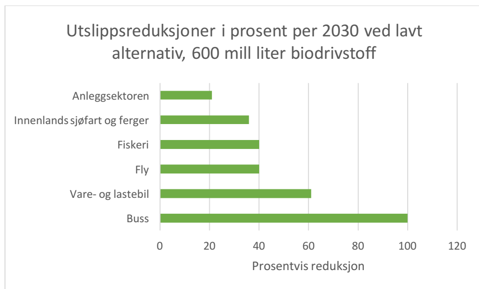
Figur 1 Næringslivet vil i våre framskrivninger i litt ulik grad klare å ta nullutslippsteknologi og gjennomføre andre tiltak for å redusere utslipp av klimagasser innen 2030.
