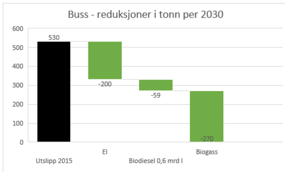
Figur 28: Bussnæringen kan bli klimanøytral allerede rundt 2030.
