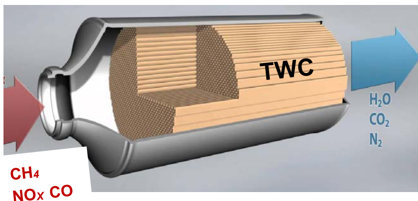
Figur 5.6: Trevegskatalysator (TWC) for rensing av avgasser fra en gassmotor. (Bilde. Hagman).
