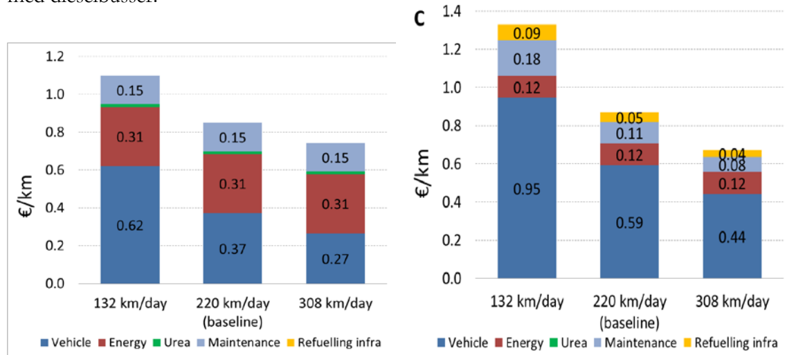
Figur 3.8: Et eksempel på kostnader for dieselbusser (til venstre) og elbusser (til høyre) per km ved ulike kjørelengde per dag (Pihlatie et al. 2014).
