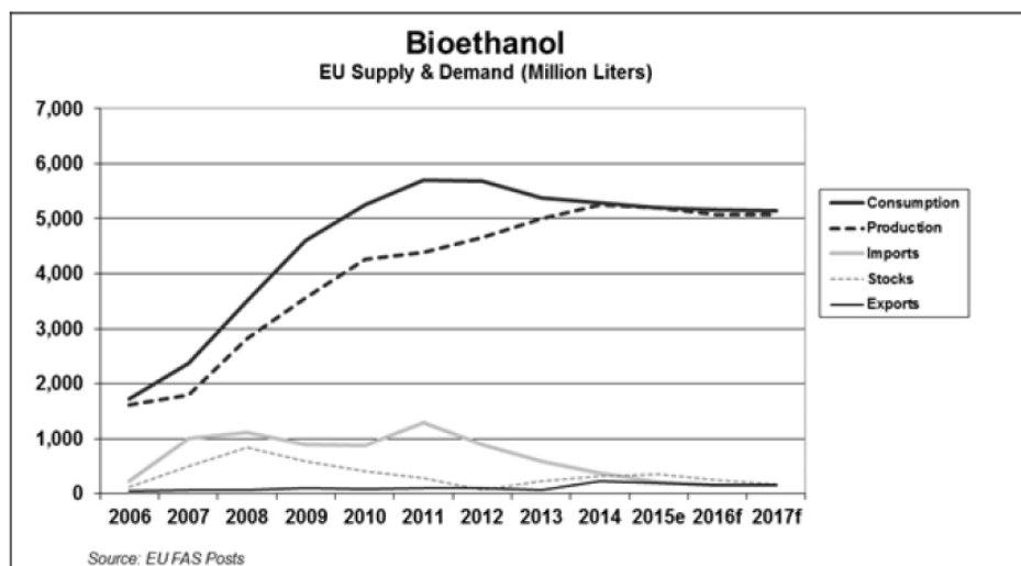
Figur 7.10: Forbruk, produksjon og import av bioetanol i EU28 i perioden 2006-2017. I mill. liter. Estimer for de siste årene. (GAIN 2016).
