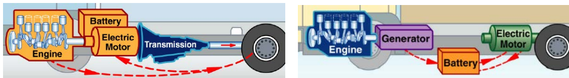
Figur 6.1: Parallell hybrid fremdrift av buss (til venstre) og seriehybrid fremdrift (til høyre). (Bilder: Southwest Research Institute).
