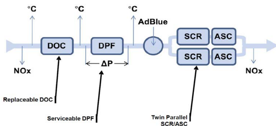
Figur 5.4: Rensesystem for rensing av dieselavgasser. Rensesystemet består av oksidasjonskatalysator "DOC", partikkelfilter "DPF", AdBlue-tilsetning, katalysator for kjemisk reduksjon av \text{NO}_x "SCR" og katalysator for fjerning av ammoniakk "ASC". (Kilde: Scania).
