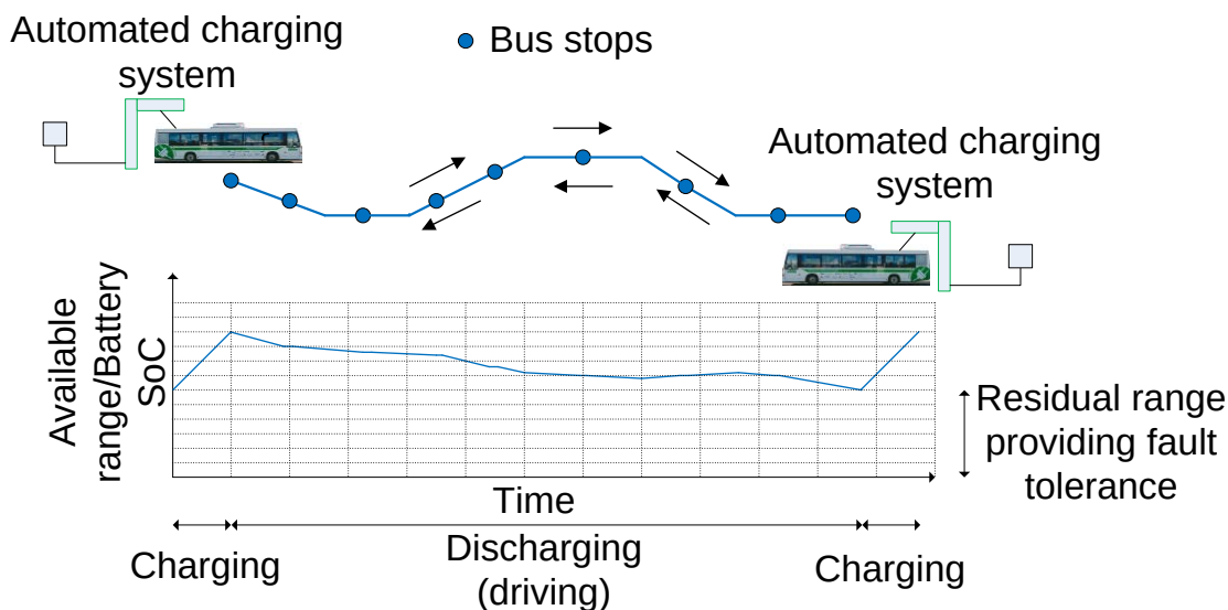
Figur 3.7: Skjematisk en bybussrute med elbusser og hurtigladning ved endestasjonene (Pihlatie et al. 2014).
