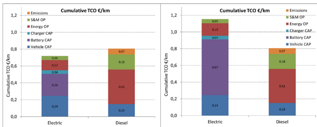
Figur 3.9: Samlede kostnader for hurtigladete busser (til venstre) og depotladete elbusser (til høyre) sammenliknet med dieselbusser på en og samme busslinje. TCO – Total Costs of Operation. (Pihlatie et al. 2016).
